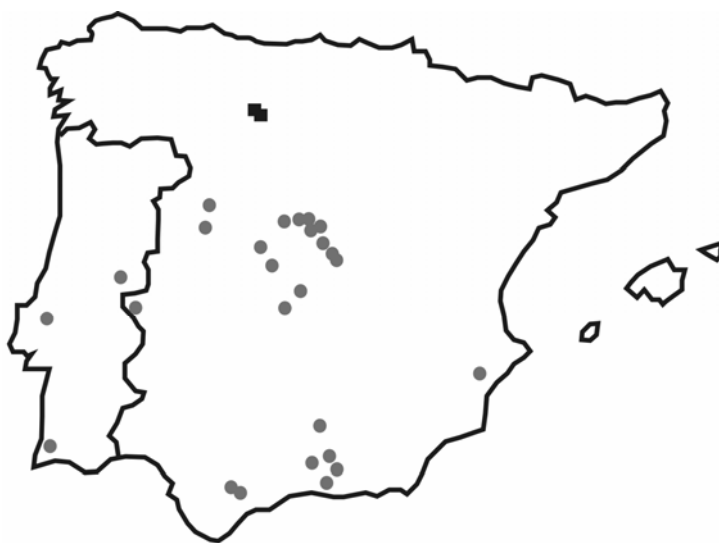
Fig. 1. Distribución de Leptynia (Leptyniella) attenuata (Pantel, 1890)
