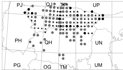
Ochloides venata
