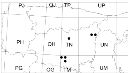
Carcharodus baeticus
