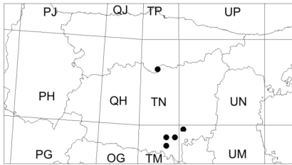
Muschampia proto
