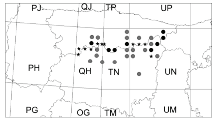
Pyrgus serratulae
