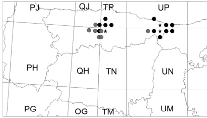
Heteropterus morpheus
