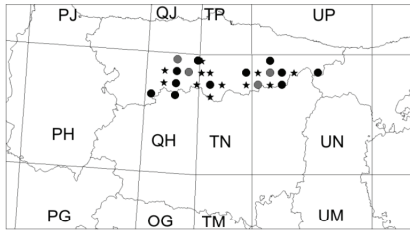
Carterocephalus palaemon
