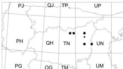
Pyrgus cirsii
