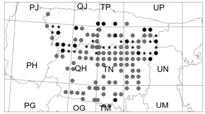
Thymelicus sylvestris
