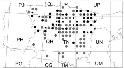
Pyrgus malvoides
