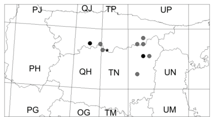
Carcharodus flocciferus
