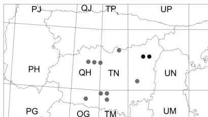
Pyrgus onopordi
